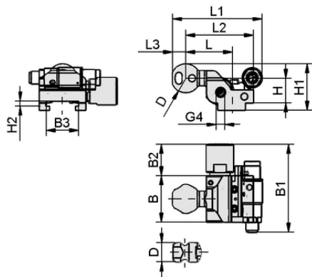
Design data HT-SG A2 I 10 46 RA AV
