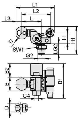
设计参数 HT-SG A2 I 10 31 G3/8-AG AV VS
