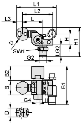
Design data HT-SG A2 I 10 31 NPT3/8-AG AV
