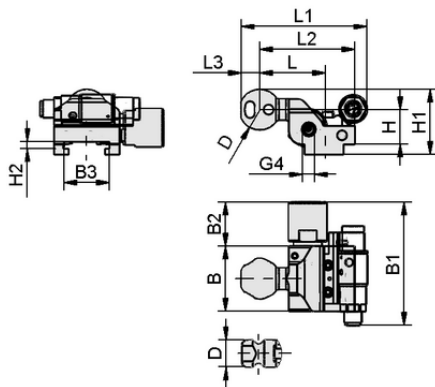
设计参数 HT-SG A3 I 10 46 RA AV VS
