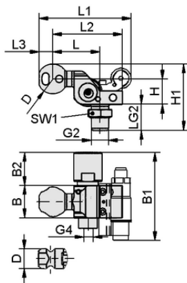
设计参数 HT-SG A3 I 10 31 G3/8-AG AV
