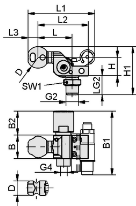
设计参数 HT-SG A5 I 10 31 G3/8-AG AV
