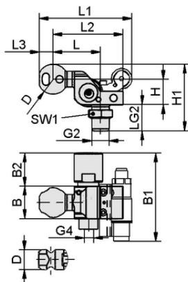
Design data HT-SG A5 I 10 31 NPT3/8-AG AV
