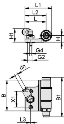
设计参数 SET HT-SG..E VSi-HD M4x12
