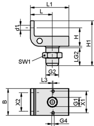
设计参数 HP-SG 2M6 E 35 G3/8-AG
