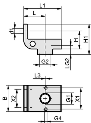
设计参数 HP-SG 2M6 E 35 G1/4-IG
