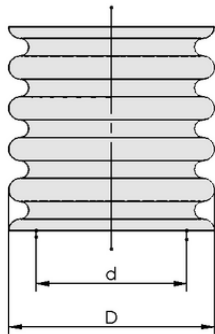
设计参数 VSL 111-100 PU-DS-AS TR
