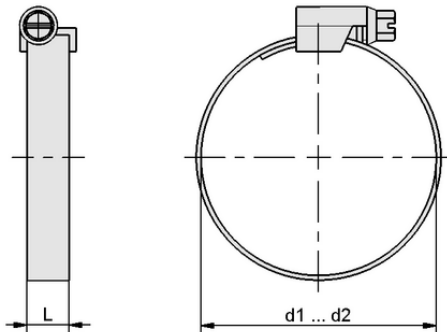
设计参数 SSB 12-20 ST-VZ
