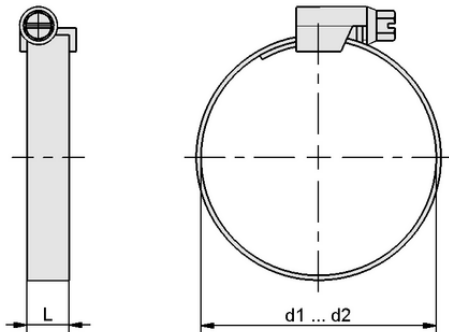
设计参数 SSB 23-35 ST-VZ
