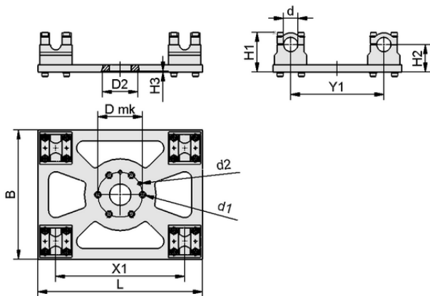
设计参数 SXT-RF-CL-D-125-40
