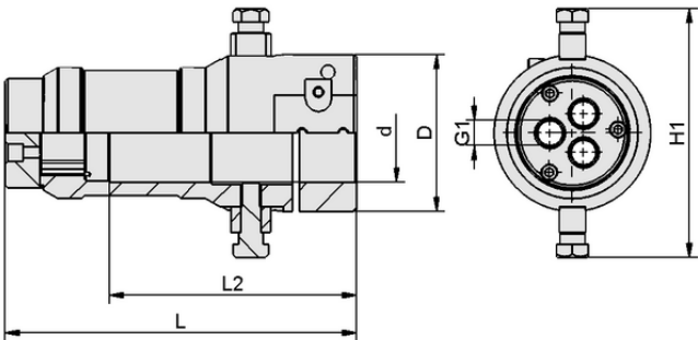
设计参数 SXT-QC-CON-60-M-6
