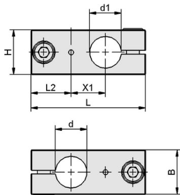
设计参数 SXT-CL X FIX 40 40 AL
