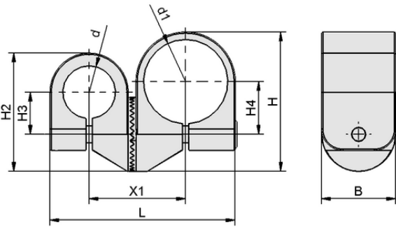
设计参数 SXT-TC-F4-0-M4
