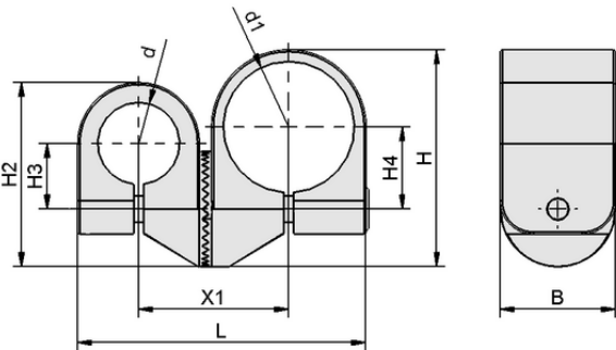
设计参数 SXT-TC-F4-0-C4
