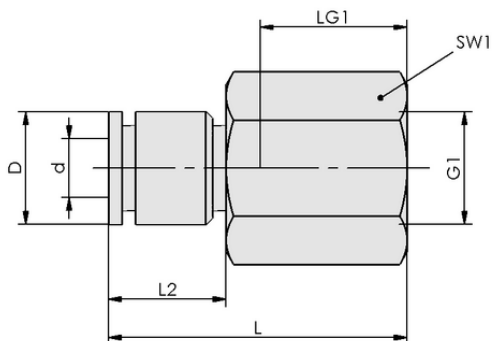
设计参数 STVI-GE G1/4-IG 4
