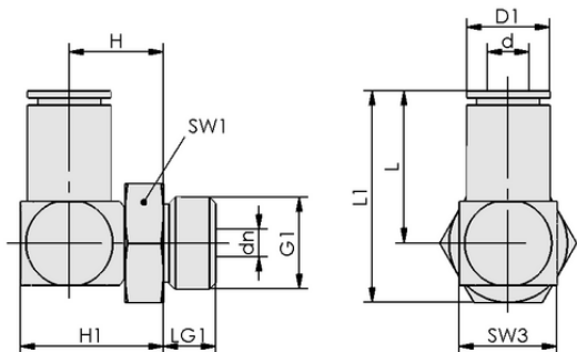
设计参数 STV-W M5-AG 4
