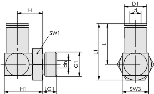
设计参数 STV-W G1/8-AG 4
