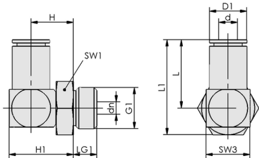
设计参数 STV-W G1/2-AG 12
