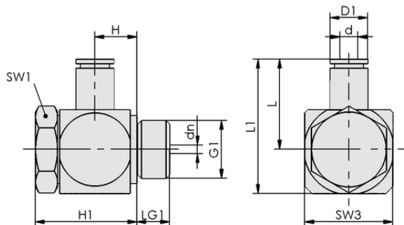
设计参数 STV-WF G1/8-AG 4
