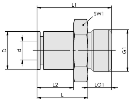
设计参数 STV-GE G1/4-AG 4
