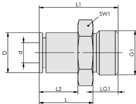
设计参数 STV-GE G1/4-AG 8
