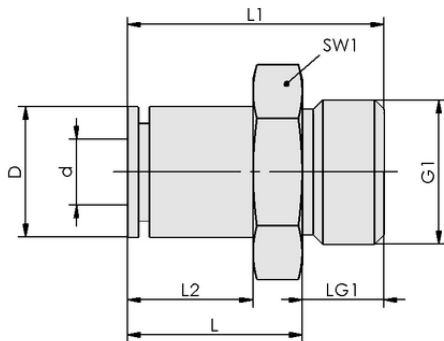
设计参数 STV-GE G3/8-AG 14
