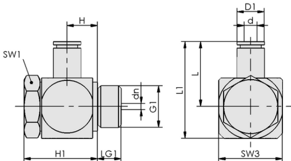
设计参数 STV-WF G3/8-AG 8
