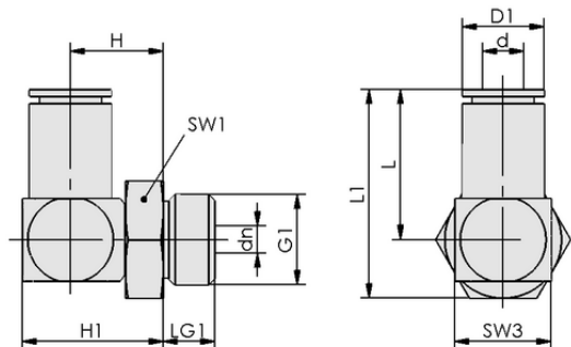
设计参数 STV-W M5-AG 6
