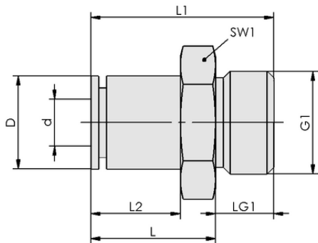
设计参数 STV-GE G3/8-AG 10
