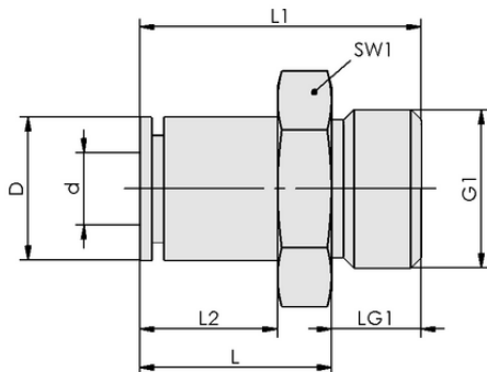
设计参数 STV-GE G1/2-AG 10
