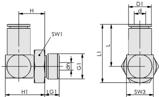
设计参数 STV-W G1/2-AG 10
