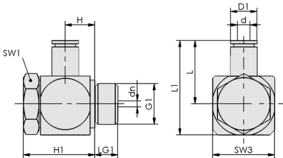
设计参数 STV-WF G3/8-AG 10
