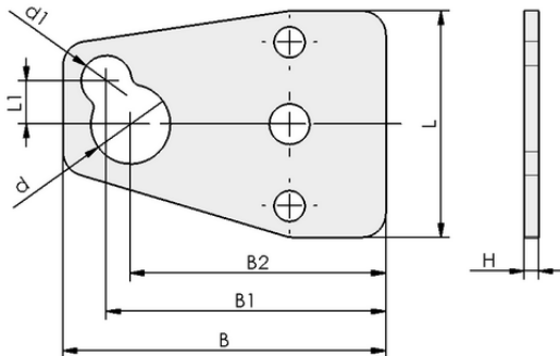
设计参数 HTR-STA 47 1N D10/16 FL
