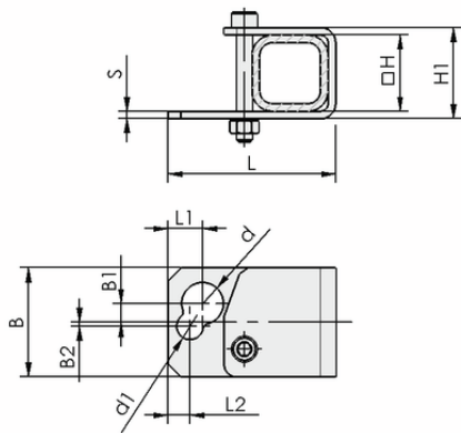
设计参数 HTR-ST5 40x40 D10/16 WI
