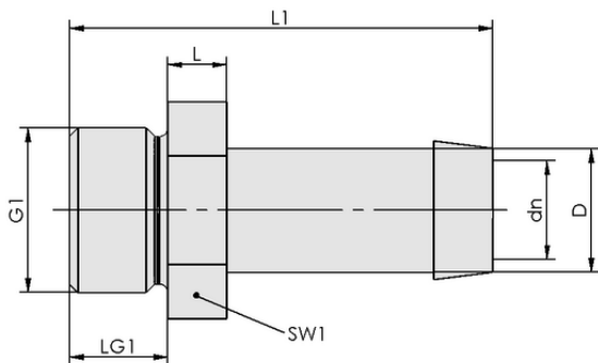
设计参数 ST M5-AG 4 MS-V
