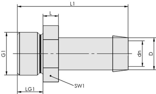
设计参数 ST G1/8-AG 6 MS-V
