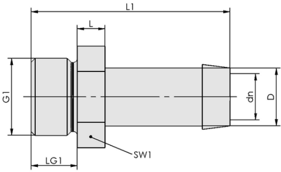
设计参数 ST G1/4-AG 6 MS-V
