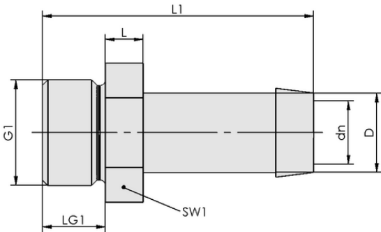
设计参数 ST G1/4-AG 13 MS-V
