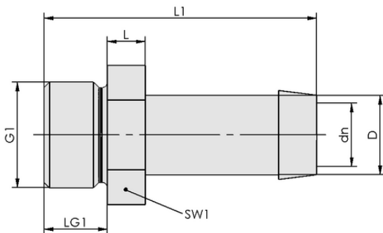
设计参数 ST G3/8-AG 9 MS-V
