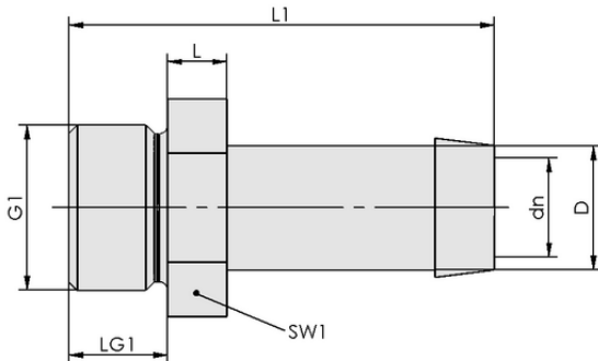
设计参数 ST G3/4-AG 19 MS-V
