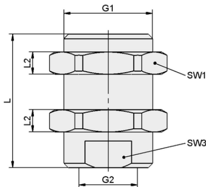
设计参数 SVS-GE M20x1.5-AG G1/4-IG 30
