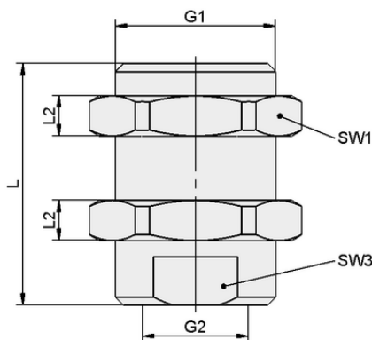
设计参数 SVS-GE M20x1.5-AG G3/8-IG 30
