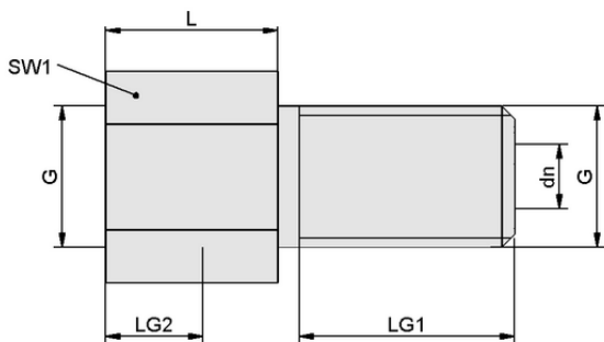
设计参数 VRL-S M5x8 MS-V
