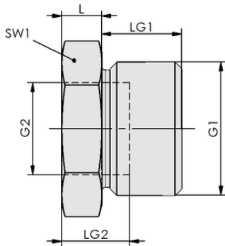
设计参数 RED-STK G1-AG G3/4-IG MS-V
