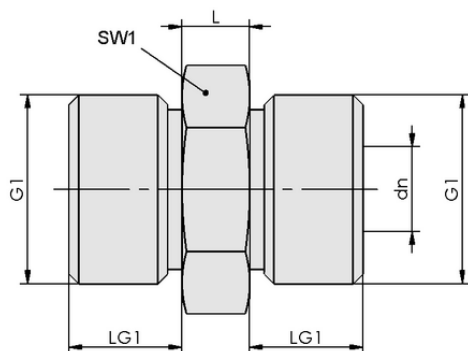
设计参数 DOP-NIP-S G1/4-AGx5
