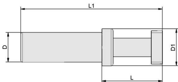
设计参数 VRS-STECH 8x18.5
