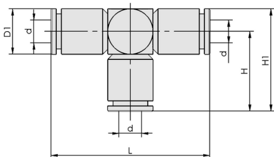
设计参数 SVB-T 10
