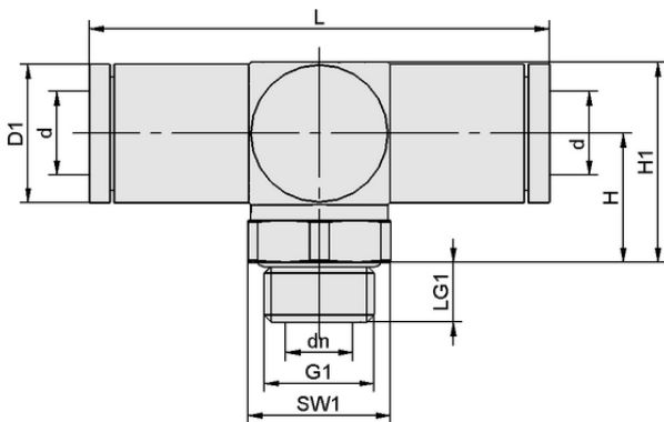
设计参数 STV-T G1/4-AG 10
