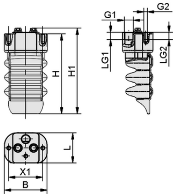
设计参数 FINGER-MODULE-2C-B-AL-SI-FOOD
