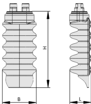
设计参数 FINGER-SPARE-UNIT 2M
